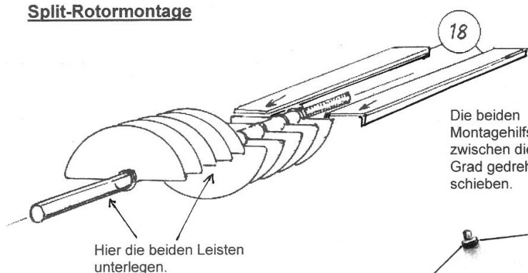
Split-Rotormontage
