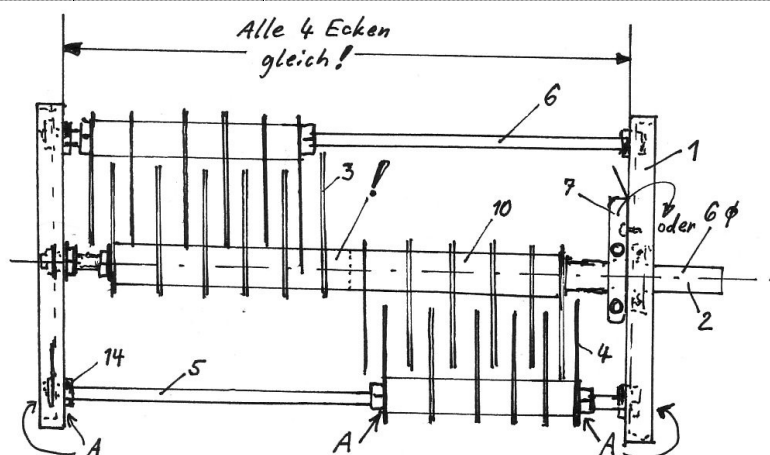
Split-Rotormontage
